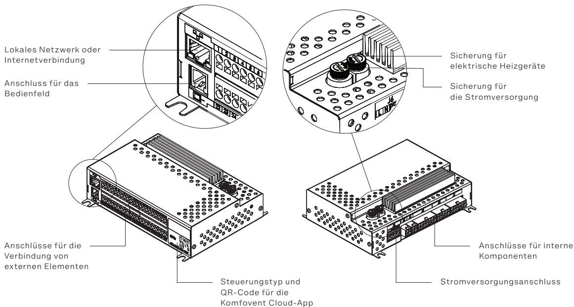
Abb. Steuerung-Hauptboard
